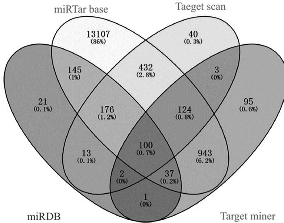
Fig. 4. Venn diagram
